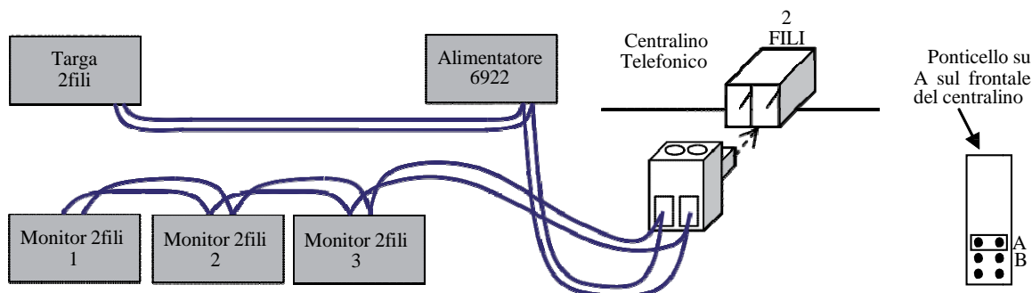
Figura 5: cablaggio dei doppino del bus Duefilel con collegamento entra-esci
