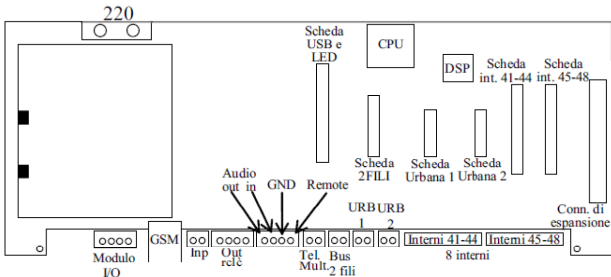
Figura 1: centralino telefonico – scheda base
