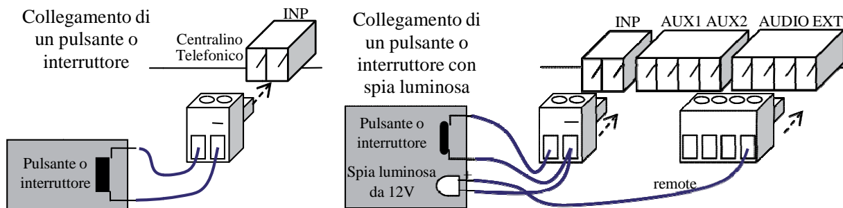
Figura 10: cablaggio dell'ingresso INP
