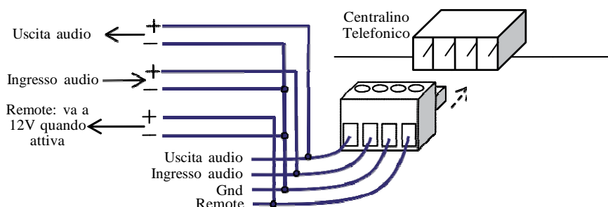
Figura 6: cablaggio dell'ingresso e uscita audio
