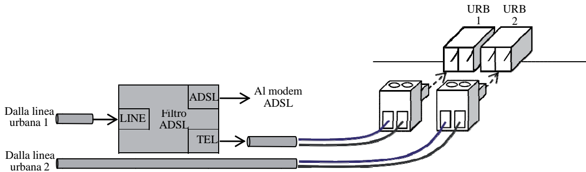
Figura 3: cablaggio dei doppini delle linee urbane
