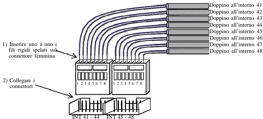
Figura 2: cablaggio dei doppi dei derivati
