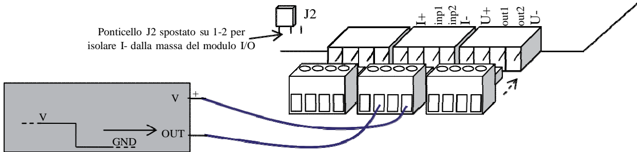
Figura 18: cablaggio dei moduli I/O – utilizzo degli ingressi con un uscita open-collector
