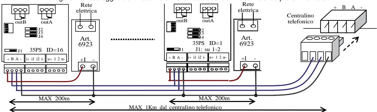
Figura 13: cablaggio dei moduli I/O – distribuzione dei moduli I/O su più alimentatori
