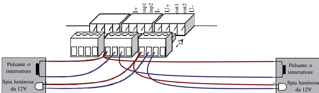
Figura 16: cablaggio dei moduli I/O – utilizzo degli ingressi con interruttore o pulsante
