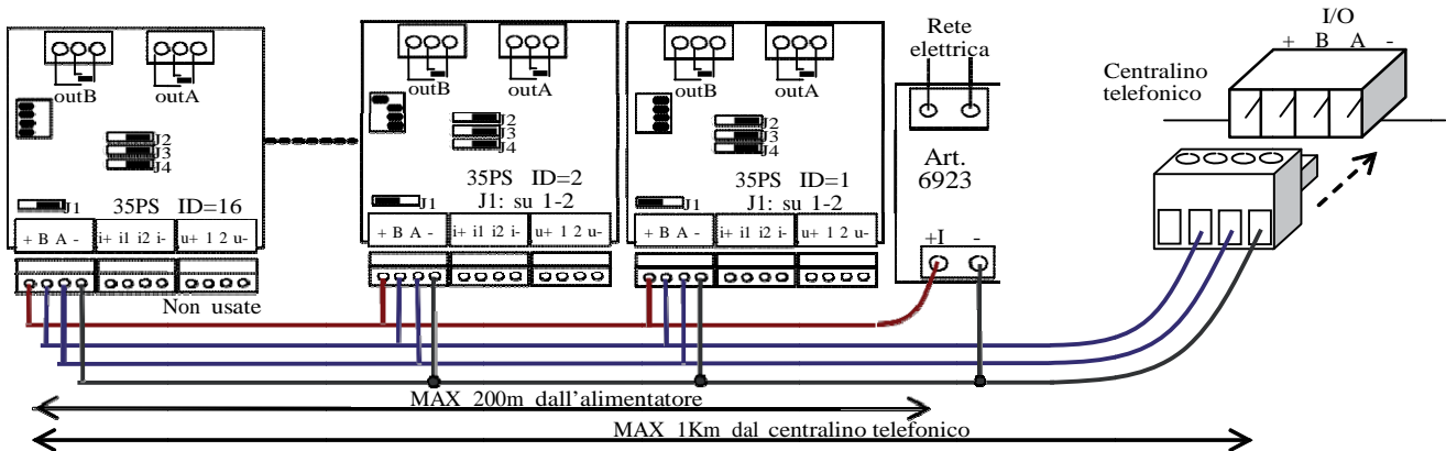
Figura 12: cablaggio dei moduli I/O – fino a 16 moduli con un unico alimentatore
