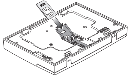
2. Einlegen der SIM-Karte
