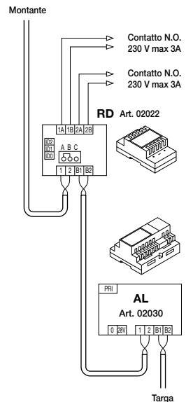
Figura 13 - Accensione luci scale con SERVIZIO AUX 1/2
