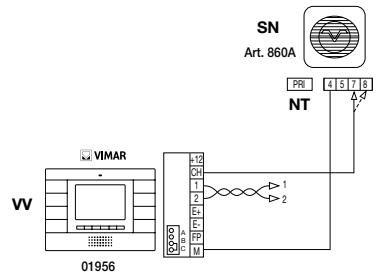
Figura 18 - Installazione con suoneria esterna Elvox
