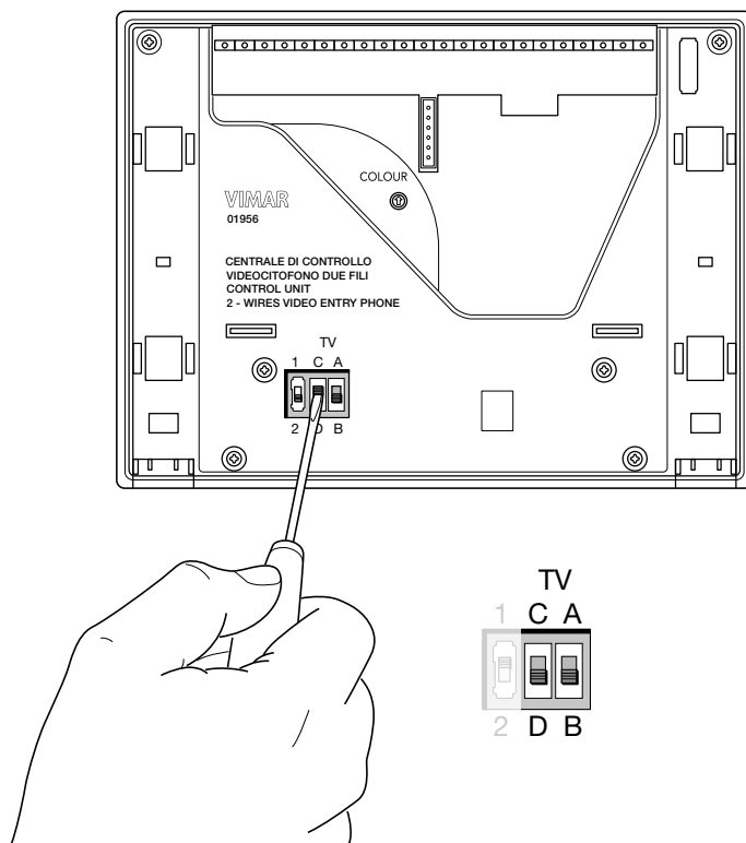
Figura 4 - Selettore di terminazione linea "TV"
