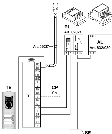
Figura 11 - Elettroserratura 15Vac 2A max
