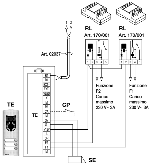
Figura 12 - Accensione luci scale con FUNZIONE F1/F2
