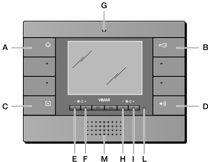
Figura 3 - Vista frontale videocitofono 01956
