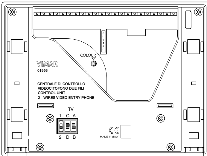
Figura 2 - Vista posteriore della centrale con videocitofono 01956
