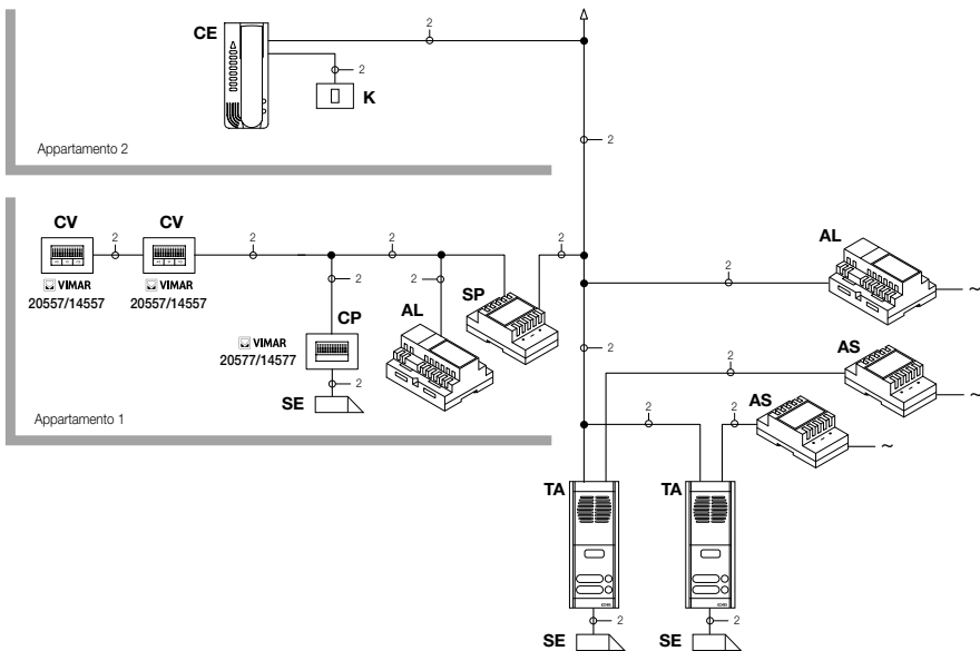
Figura 24 - Chiamata fuori porta solo audio
