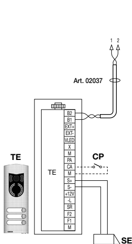
Figura 10 - Elettroserratura 12Vcc 200mA max
