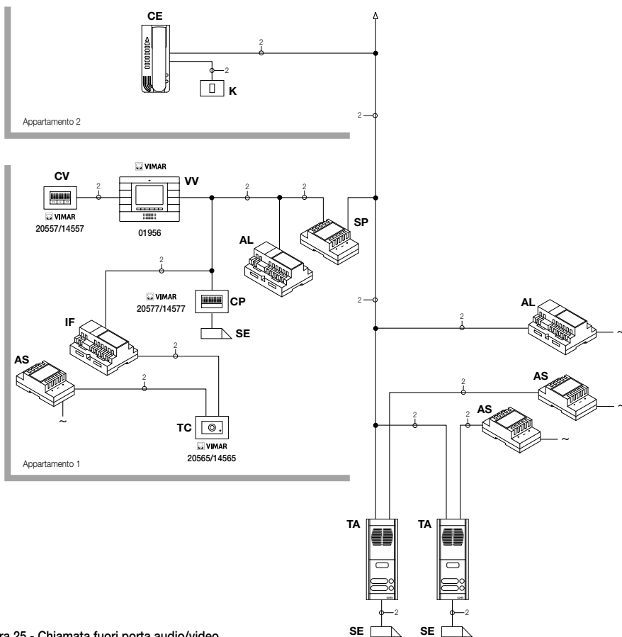
Figura 25 - Chiamata fuori porta audio/video
