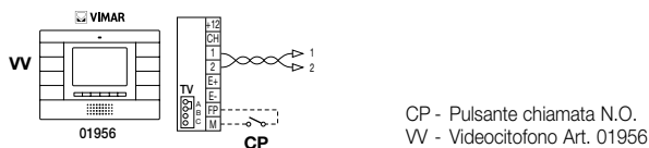
Figura 14 - Chiamata da campanello
