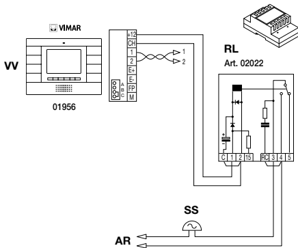
Figura 17 - Installazione suoneria esterna con relè
