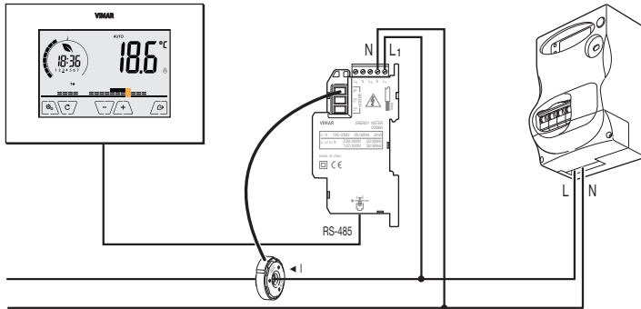
Fig. 2: Configuración básica para la medición de la absorción doméstica
