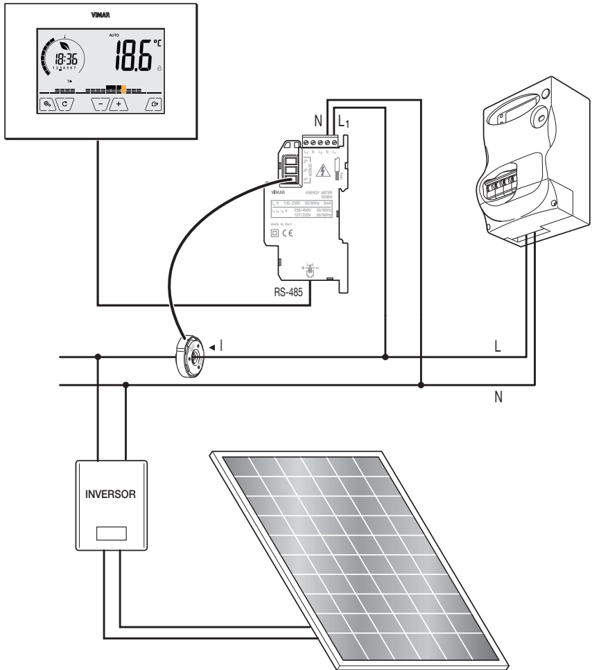
Fig. 4: Medición del consumo neto o de la producción de la instalación fotovoltaica. En caso de producción con paneles fotovoltaicos (con cesión a la compañía eléctrica), la sonda registra un valor NEGATIVO que corresponde a una producción energética (lo contrario de un consumo).
