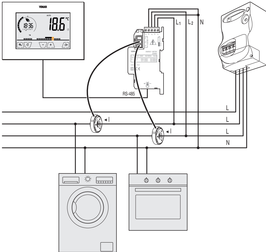
Fig. 3: Medición del consumo global de una instalación, también con cargas (monofásicas) distribuidas en distintas fases.
