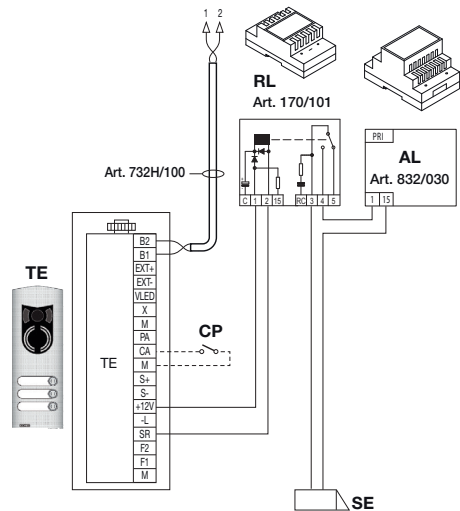
Figura 5 - Elettroserratura 15Vac 2A max
