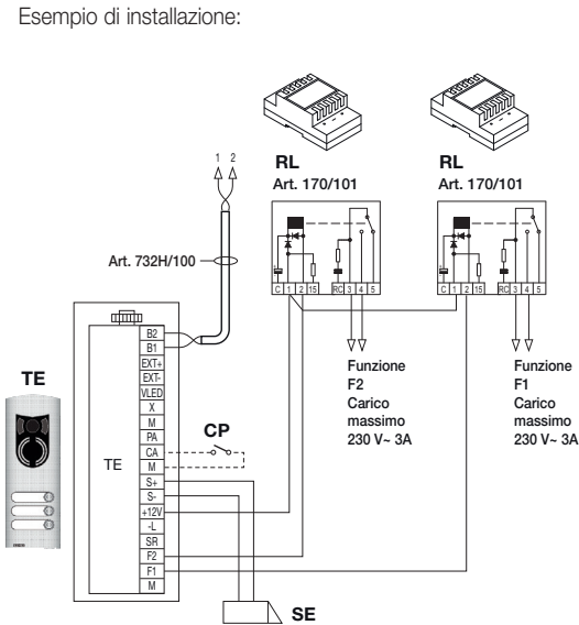
Figura 6 - Accensione luci scale con FUNZIONE F1/F2
