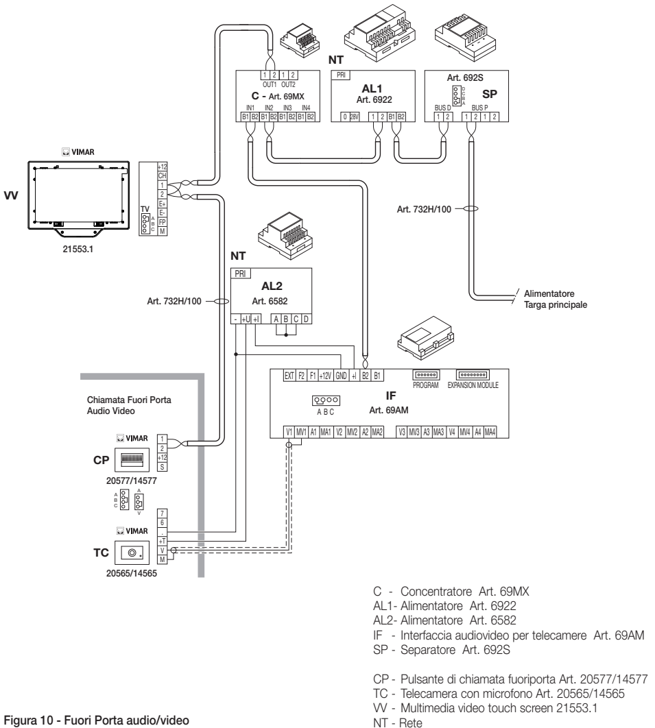
Figura 10 - Fuori Porta audio/video
