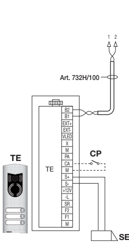
Figura 4 - Elettroserratura 12Vcc 200mA max
