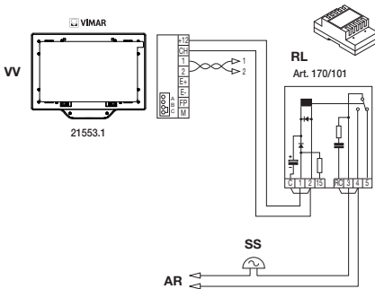
Figura 11 - Installazione suoneria esterna con relé
