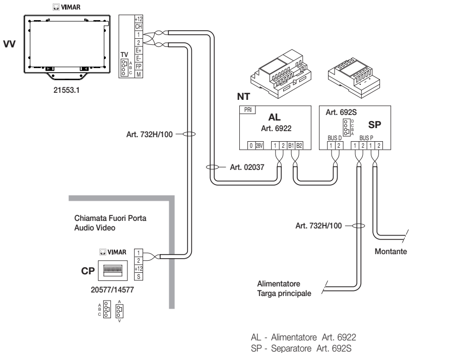
Figura 9 - Fuori Porta solo audio
