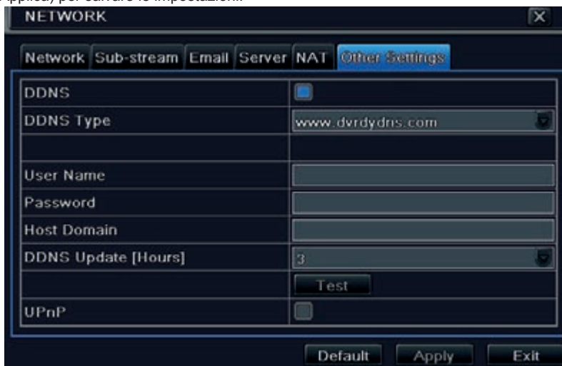
Fig. 4-27 Configurazione di rete - Altre impostazioni
