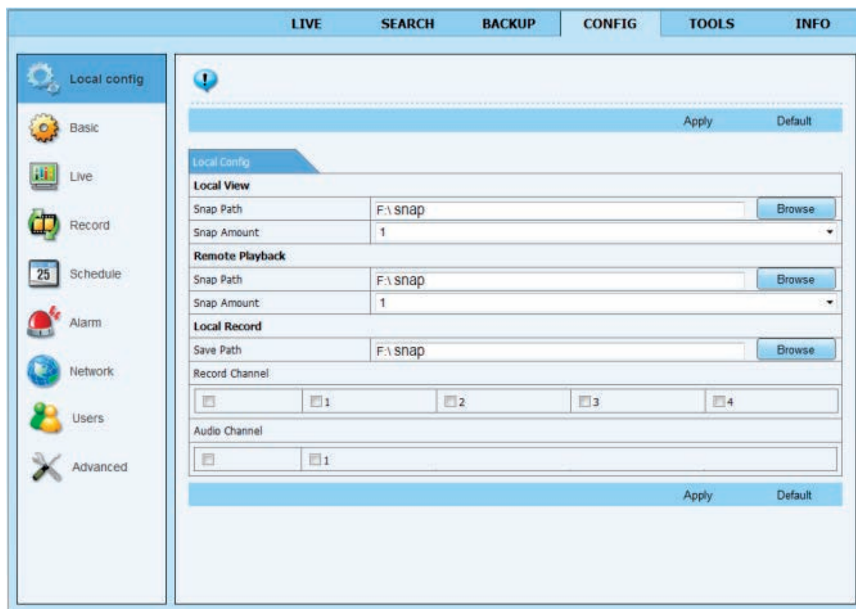
Fig. 7-9 Configurazione dei menu in remoto
