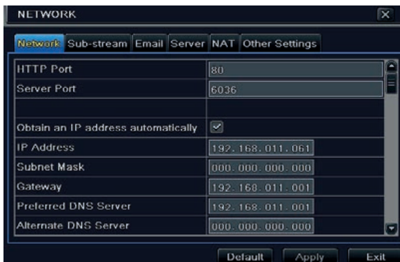
Fig. 4-22 Configurazione di rete - Rete
