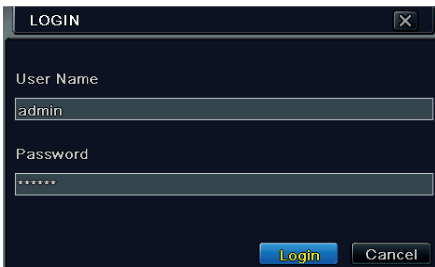
Fig. 3-1 Login
