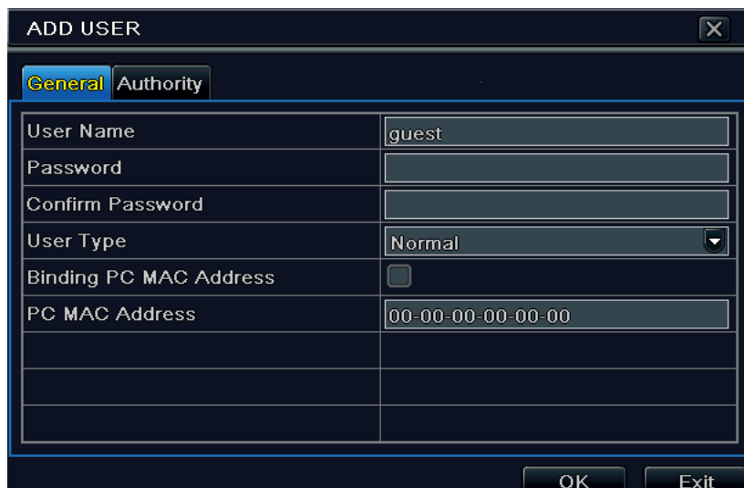
Fig. 4-30 Aggiungi - Generale
