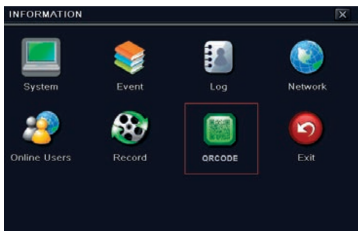
Fig. 6.-1 Configurazione informazioni
