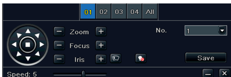
Fig. 4-35 Configurazione preimpostazioni
