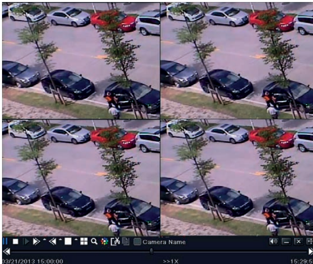
Fig. 3-3 Riproduzione Live
