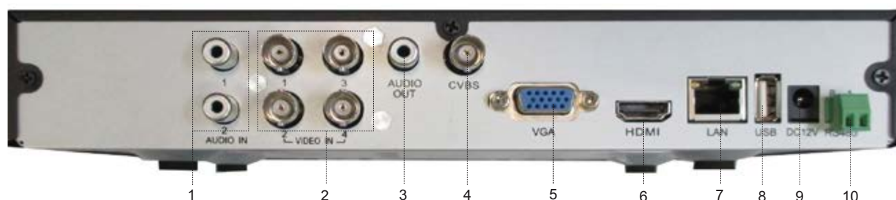
Fig. 2-1 Pannello posteriore 4-CH
