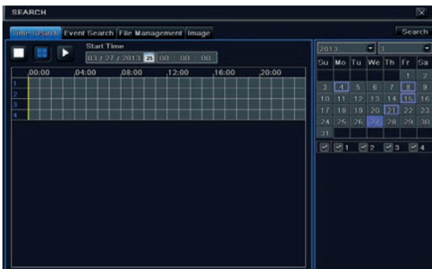
Fig. 5-1 Configurazione della ricerca - Ricerca cronologica
