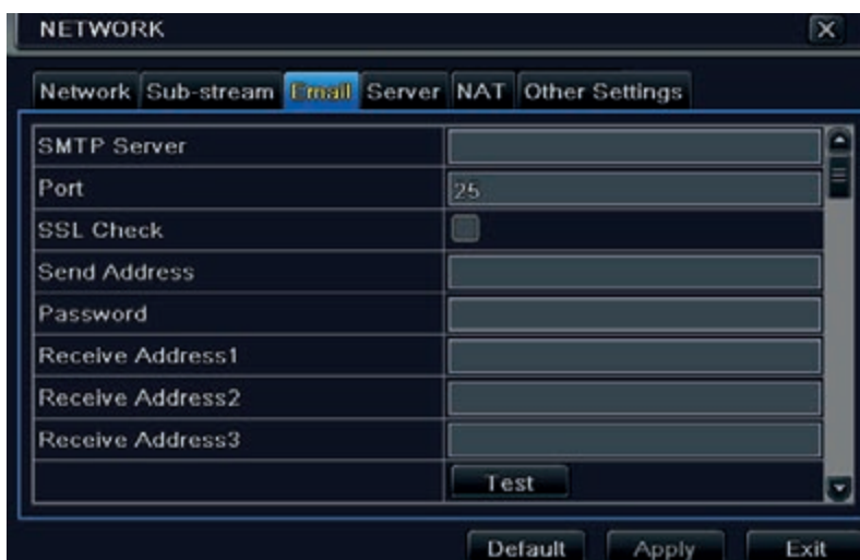
Fig. 4-24 Configurazione di rete - Email
