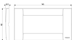
Vista ingombri
